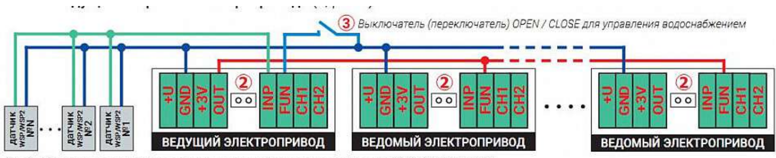
Рис. 1. Объединение в систему нескольких шаровых электроприводов из серий GIDROLOCK WINNER
